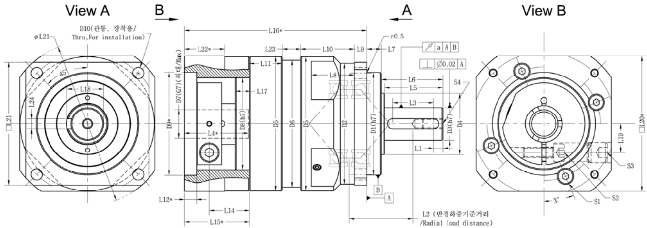
CA C2 输入方式尺寸表 CA C2 input style Dimensions (mm)
