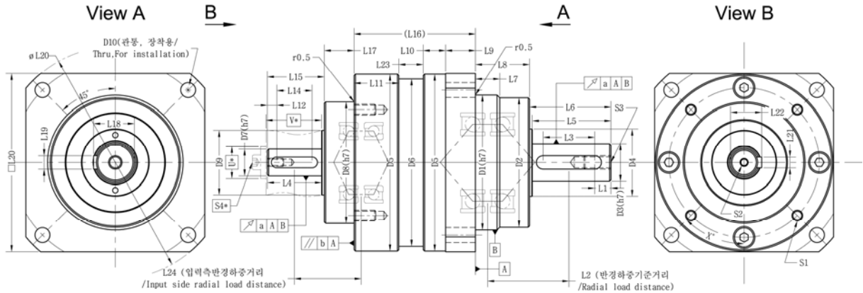
CP S2 输入方式尺寸表 CP S2 input style Dimensions (mm)
