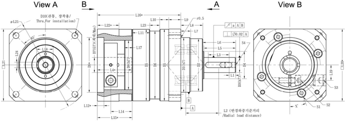
CP C2 输入方式尺寸表 CP C2 input style Dimensions (mm)
