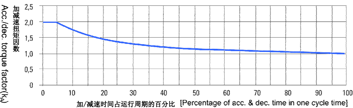
CP 系列 加/减速扭矩因数图表 CP series Acceleration/Deceleration torque factor diagram
