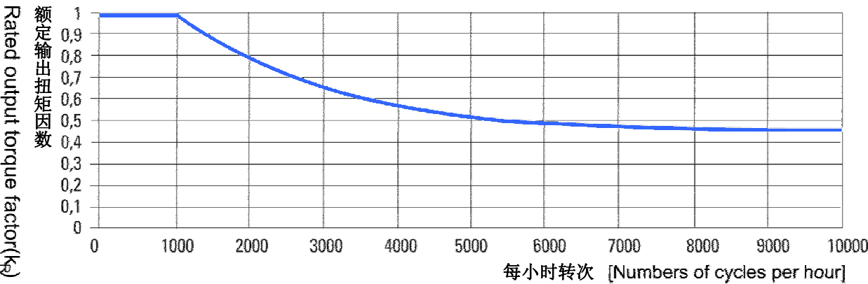
CP 系列 额定输出扭矩因数图表 CP series rated output torque factor diagram
